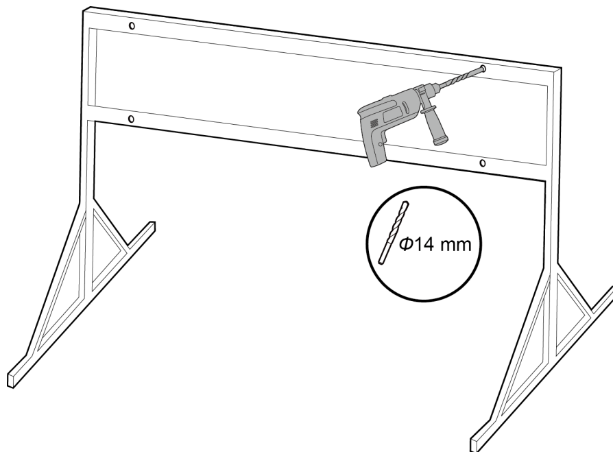
Figura 4-11 Cómo perforar un orificio
