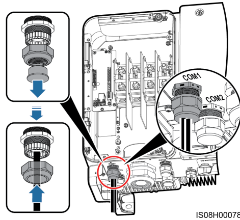
Figura 5-31 Tendido de cables
