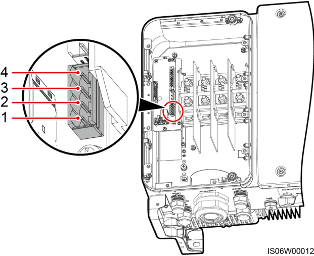
Figura 5-23 Regleta de conexión
