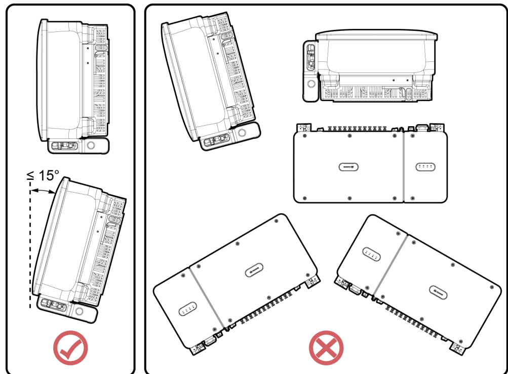
Figura 4-4 Posición de instalación
