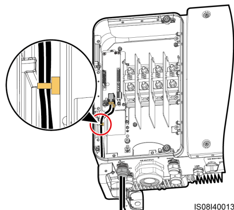
Figura 5-33 Agrupación de los cables de comunicaciones
