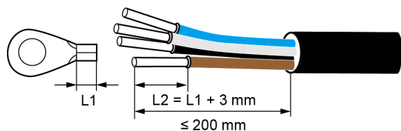
Figura 5-11 Cable de cuatro núcleos (excluye el cable de tierra pero incluye el conductor neutro)
