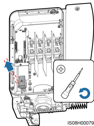
Figura 5-35 Cómo retirar la cubierta de protección
