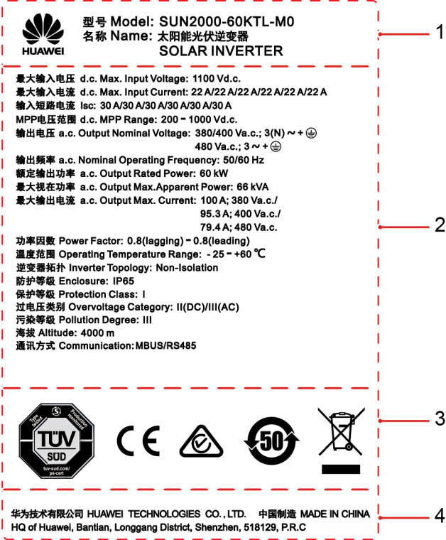
Figura 2-4 Placa de identificación del SUN2000-60KTL-M0
