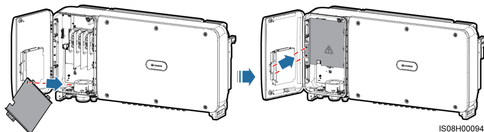
Figura 5-40 Instalación de la tapa
