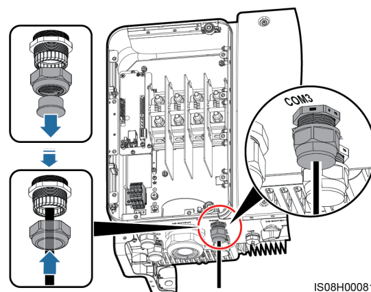
Figura 5-36 Tendido de cables
