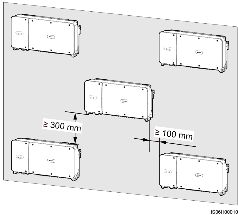
Figura 4-6 Modo de instalación triangular (recomendado)
