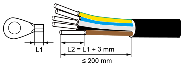
Figura 5-12 Cable de cinco núcleos (incluye el cable de tierra y el conductor neutro)
