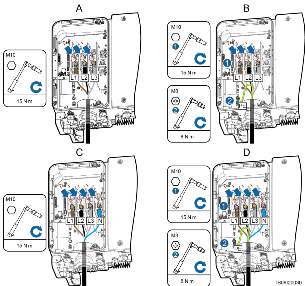
Figura 5-13 Conecte el cable de alimentación de salida de CA del SUN2000-50KTL/60KTL-M0
