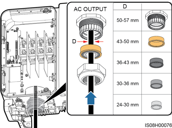
Figura 5-8 Tendido de cables
