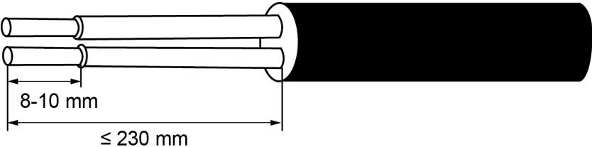
Figura 5-24 Cómo pelar un cable de comunicaciones RS485
