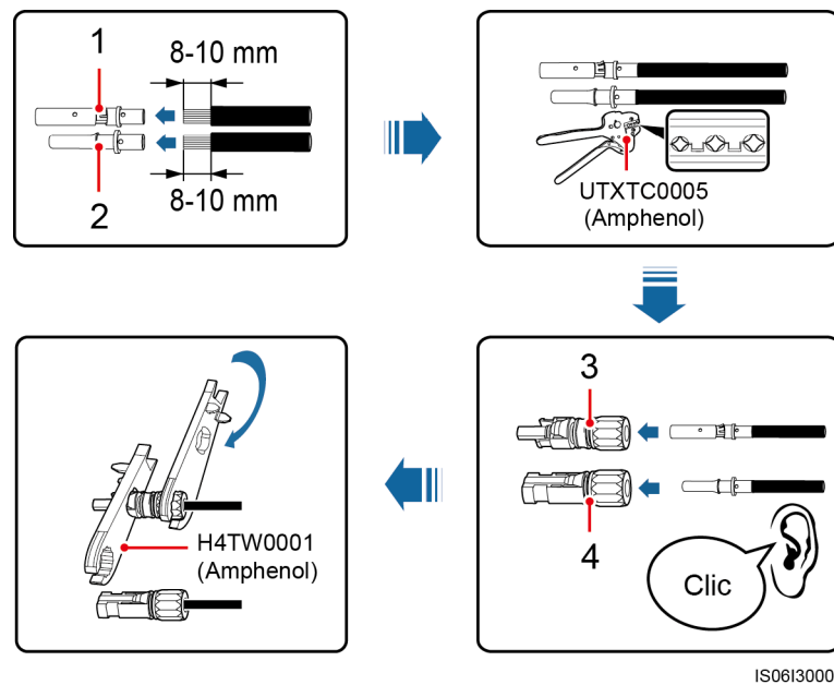
Figura 5-17 Preparación de los conectores positivo y negativo (utilizando contactos metálicos de conformado en frío).
