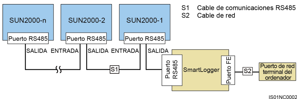
Figura 5-22 Modo de comunicación para múltiples SUN2000
