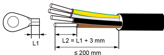
Figura 5-10 Cable de cuatro núcleos (incluye el cable de tierra pero no el conductor neutro)
