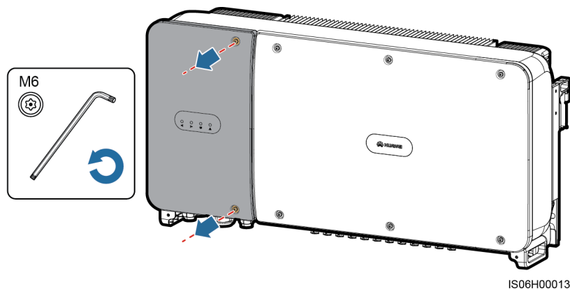
Figura 5-3 Desajuste de tornillos
