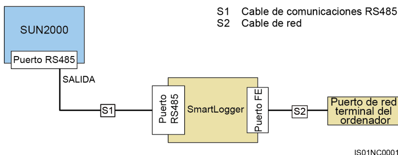
Figura 5-21 Modo de comunicación de un solo SUN2000
