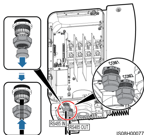
Figura 5-25 Tendido de cables
