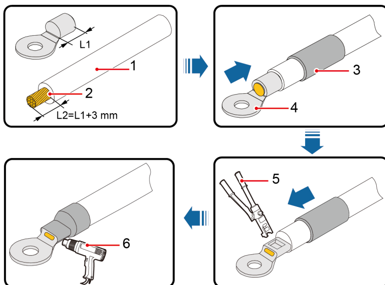
Figura 5-2 Engaste del terminal OT
