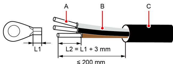
Figura 5-9 Cable de tres núcleos (excluye el cable de tierra y el conductor neutro)
