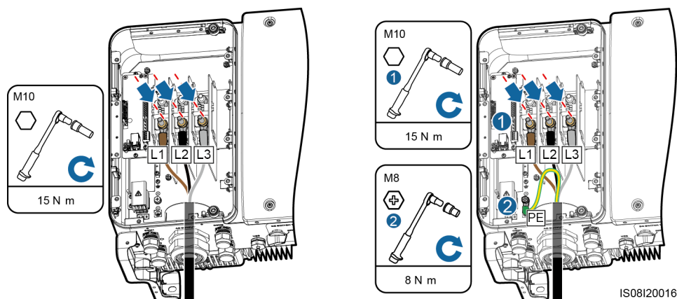
Figura 5-14 Conecte el cable de alimentación de salida de CA del SUN2000-65KTL-M0
