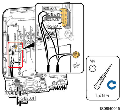
Figura 5-27 Conexión de los cables de comunicaciones
