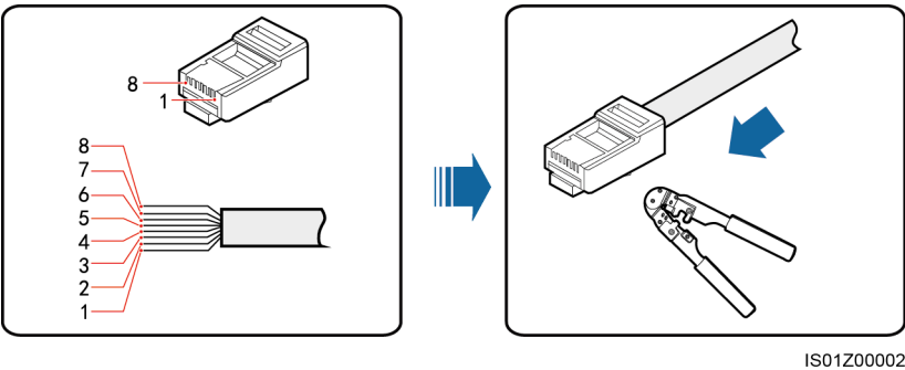
Figura 5-30 Preparación de un conector RJ45
