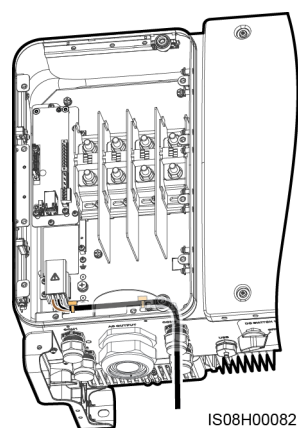
Figura 5-39 Cómo enlazar un cable de alimentación del seguidor solar
