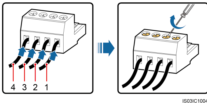
Figura 5-26 Conexión de cables a una base de terminales
