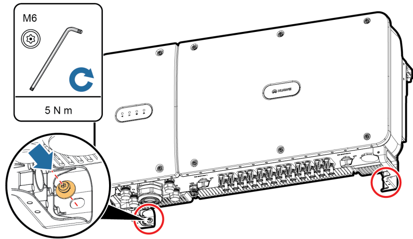
Figura 4-19 Ajuste de tornillos antirrobo
