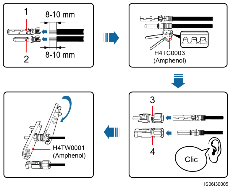
Figura 5-18 Preparación de los conectores positivo y negativo (utilizando contactos metálicos de conformado por estampado).
