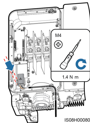
Figura 5-38 Instalación de la cubierta de protección
