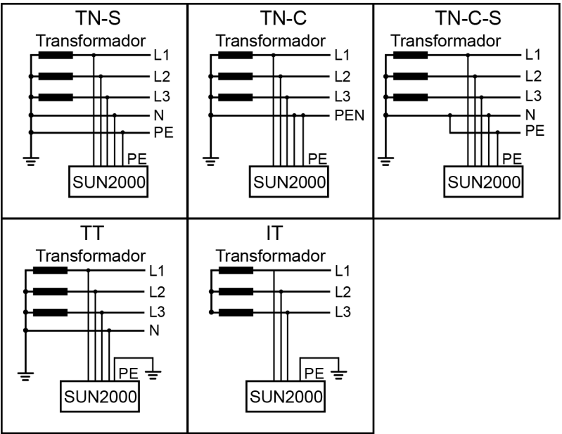
Figura 2-3 Modos de red eléctrica
