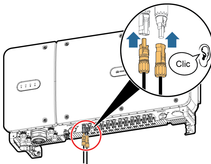
Figura 5-20 Conexión de los cables de entrada de CC
