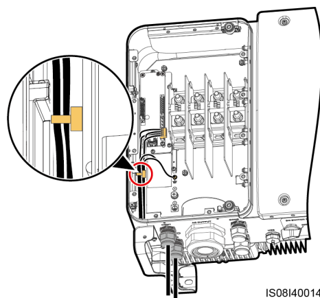
Figura 5-28 Agrupación de los cables de comunicaciones
