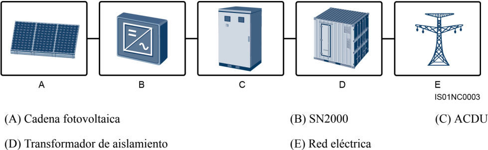
Figura 2-2 Diagrama de red
