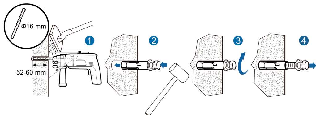
Figura 4-14 Perforación de un orificio e instalación de un perno de expansión
