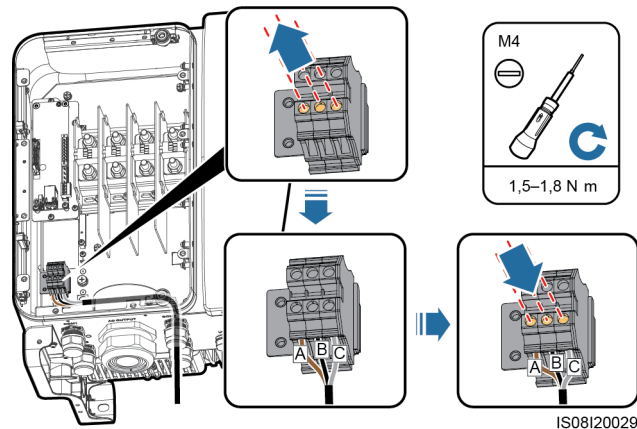
Figura 5-37 Conexión de un cable de alimentación del seguidor solar
