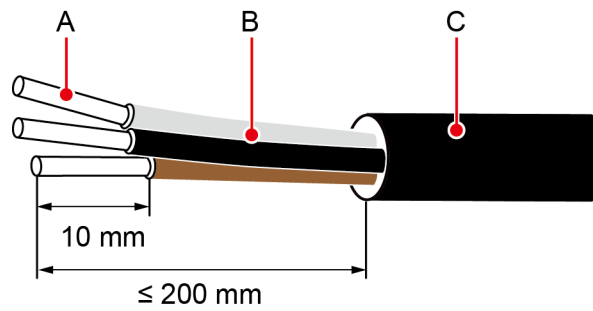
Figura 5-34 Cómo pelar un cable
