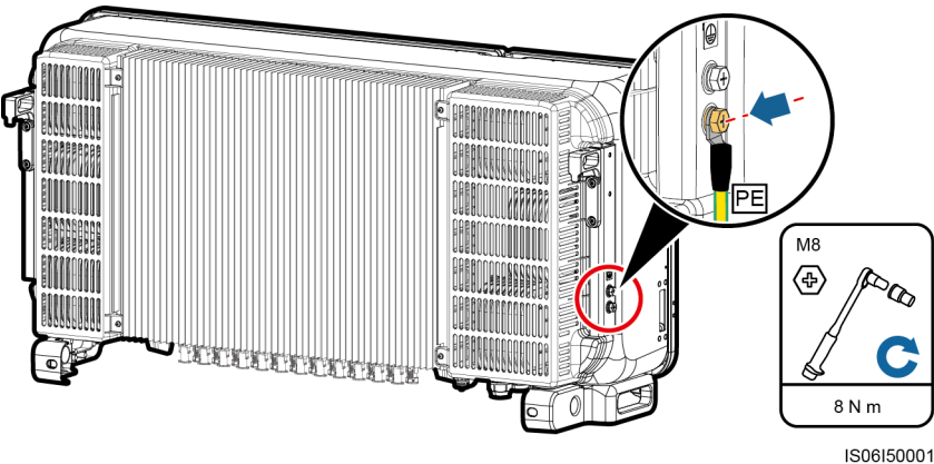
Figura 5-7 Cómo conectar un cable de tierra
