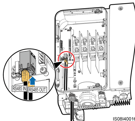
Figura 5-32 Conexión de los cables de comunicaciones
