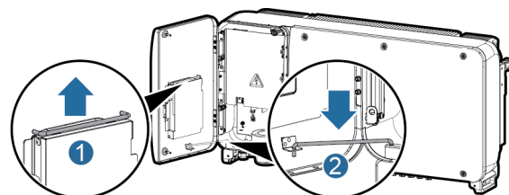
Figura 5-5 Cómo mantener la puerta abierta con la barra de soporte
