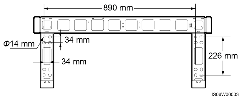
Figura 4-8 Dimensiones de la ménsula de montaje
