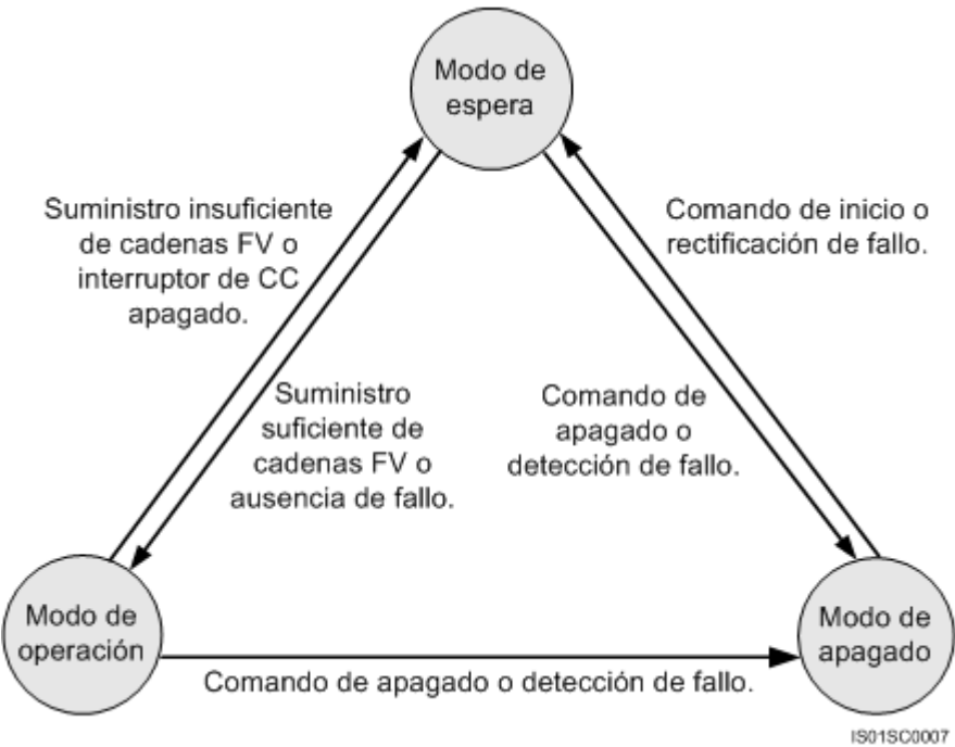
Figura 2-7 Modos de funcionamiento del SUN2000
