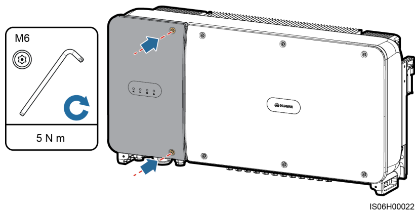
Figura 5-42 Ajuste de los tornillos
