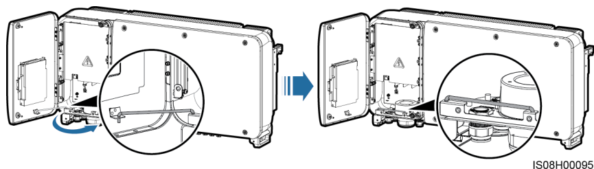
Figura 5-41 Cómo extraer la barra de soporte
