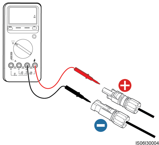
Figura 5-19 Medición de la tensión
