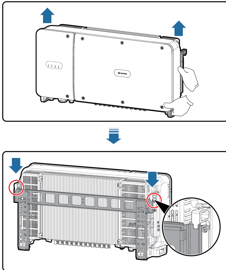
Figura 4-18 Colocación del SUN2000 en la ménsula de montaje
